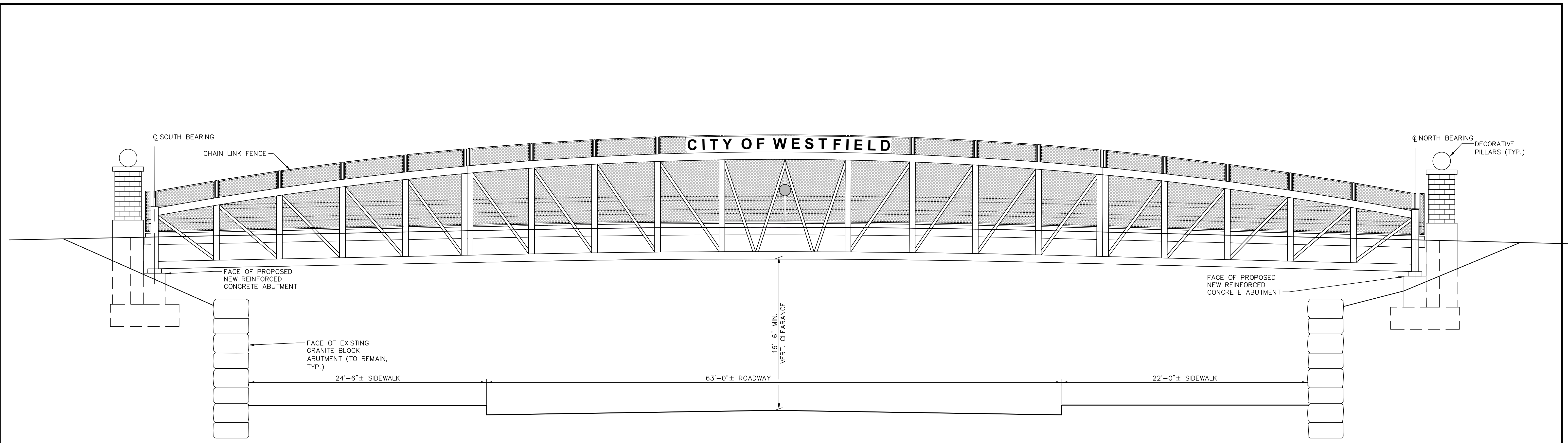
ELEVATION SCALE: 3/16" = 1'-0"
